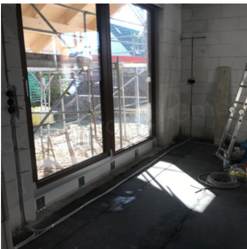
45: Verlegen der ELT-Leitungen; Abdichten BP EG
